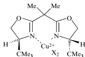
(47): X = CF 3 SO 3 -
